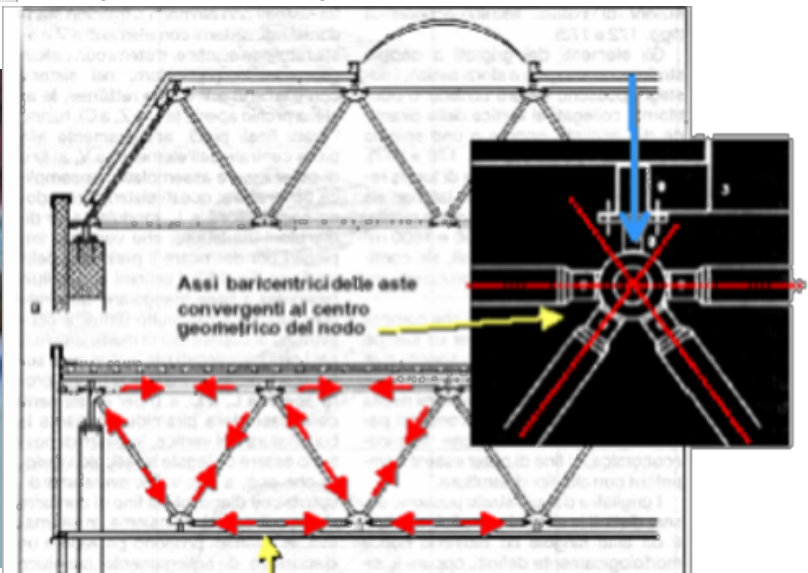
Elementi reticolari
