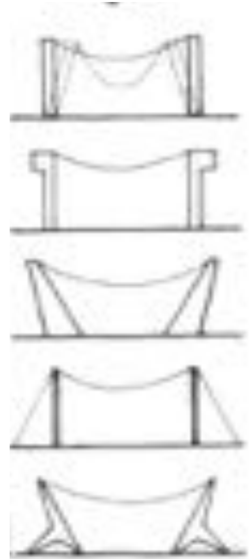
piedritti
