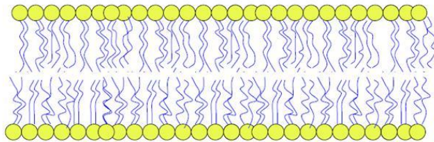
FASE LIQUIDO-CRISTALLINA
