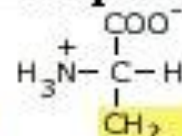
Triptofano
