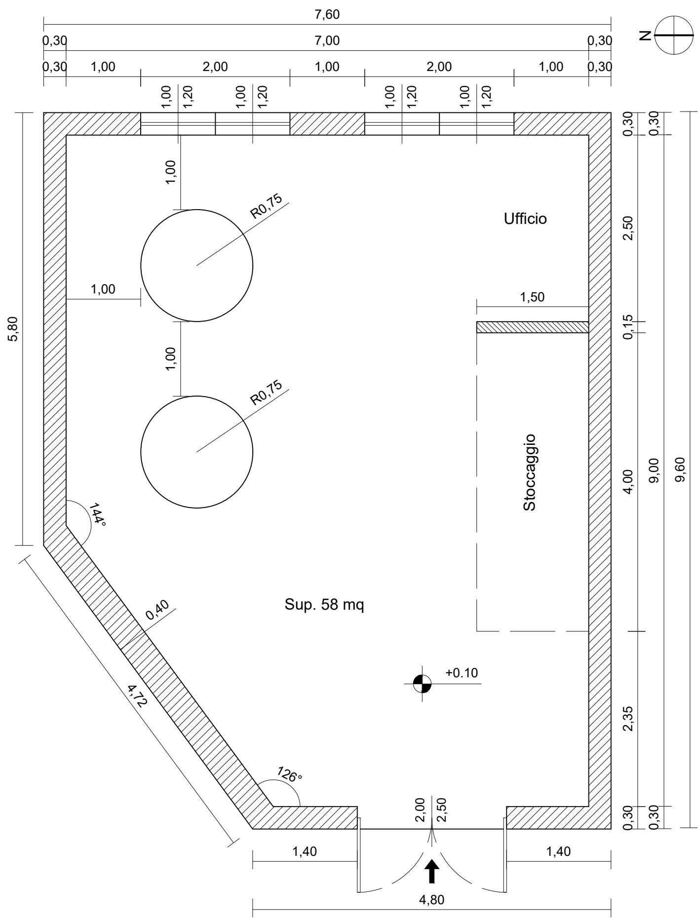
Pianta deposito
